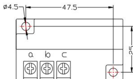
Рисунок 4.1.4. Установочные
