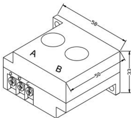
Рисунок 4.1.3. Структурные размеры
